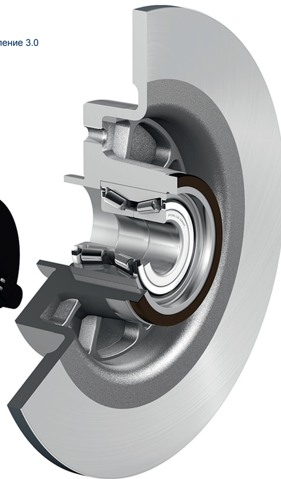
Узел ступицы колеса с интегрированным диском тормозного механизма HUB UNIT with integrated Brake disc
