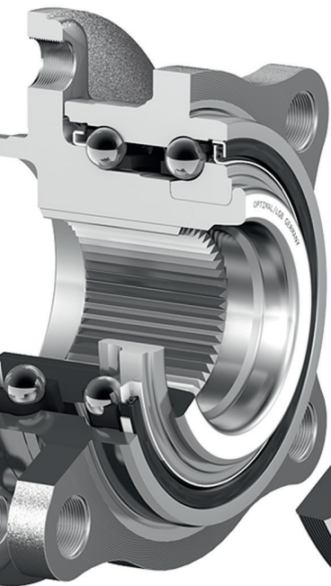
Узел ступицы колеса. Поколение 3.1 HUB UNIT Generation 3.1
